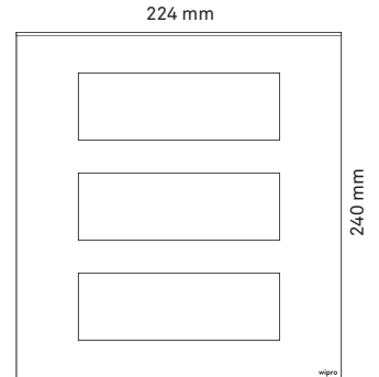
18 Module Plate
